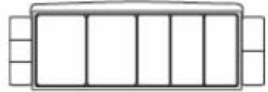
Номер позиции: BD4023S; Охлаждаемый Масса: 1,81 кг Конфигурация лотков: (2) лотка по 1,65 л, (3) лотка по 0,475л, (2) контейнера для соломинок
